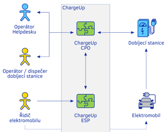
Obr. 1 - Ekosystém dobíjecí stanice
